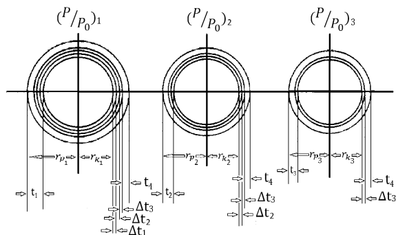
شکل ۱- طرح اجمالی کلی مکانیزم فرض شده در روش BJH [۶]
