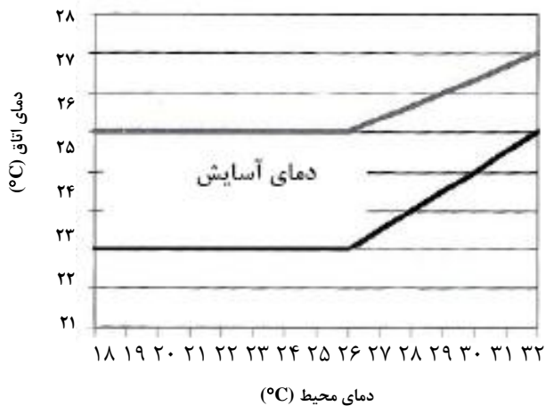
شکل ۵- نمودار دمای آسایش در ساختمان‌های مسکونی [۱۷]
