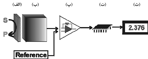
شکل ۱- طرح اجمالی حسگر زیست‌شناختی [۴]
