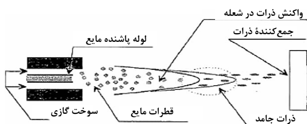
شکل ۶- طرح اجمالی روش پاشش مایع در شعله برای سنتز نانو ذرات [۲۶]
