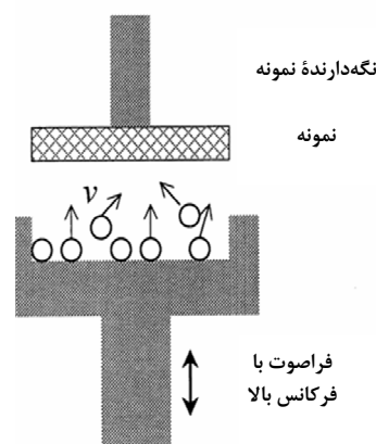
شکل ۴- طرح اجمالی روش کوبش با استفاده از امواج
