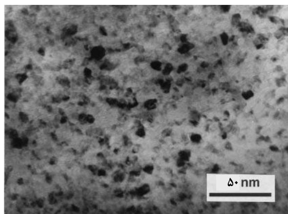
شکل ۵- تصویر TEM گرفته شده از سطح ورقه آهن
