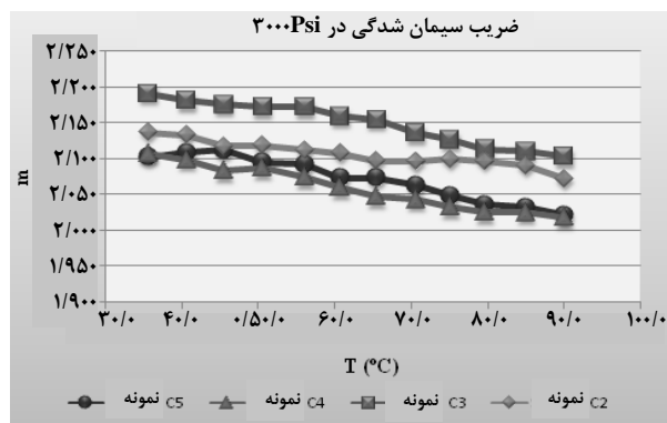
شکل ۲- مقادیر پارامتر m تحت تأثیر دما در فشار ۳۰۰۰ Psi
